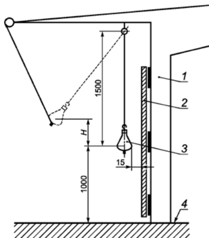
Рисунок ДА.1 - Маятник для нежесткого удара
