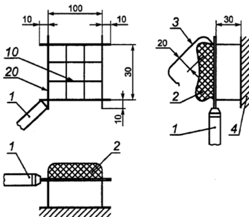
1 - ручка; 2 - ватный тампон; 3 - зажим; 4 - поверхность опытного образца
