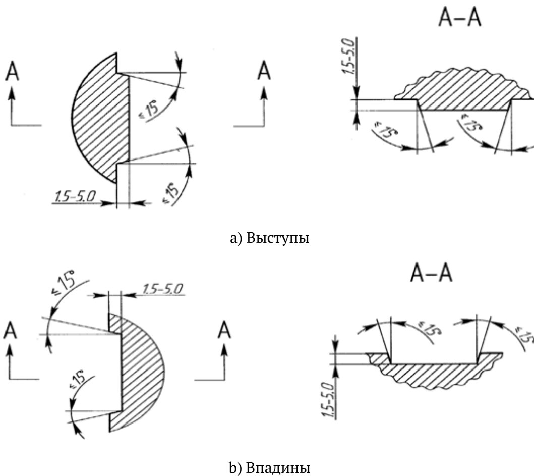
Рисунок 7. Скосы краев и впадин
