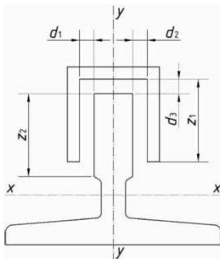
а) Номинальное положение и зазоры контрольного башмака
