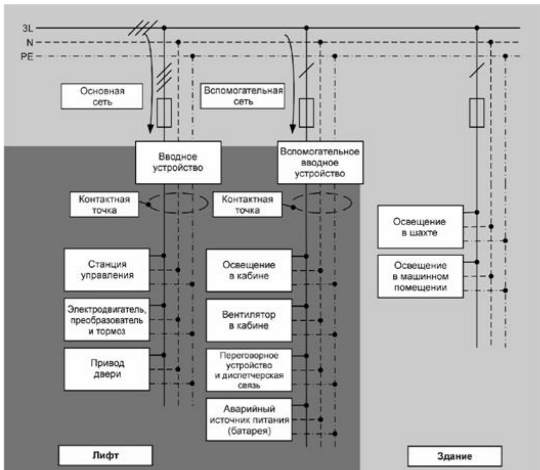
Рисунок А.1 - Подключение средств измерения энергопотребления лифтов
