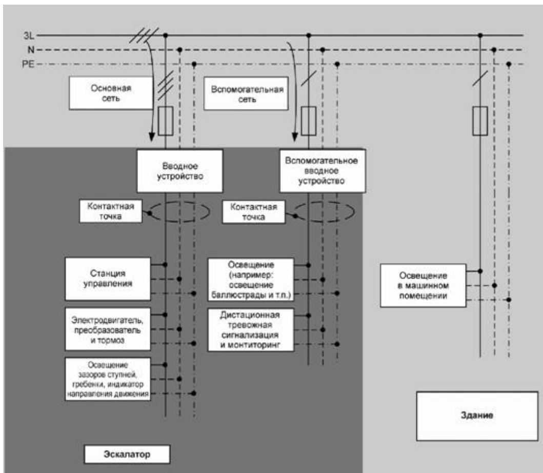
Рисунок А.2 - Подключение средств измерения энергопотребления эскалаторов
