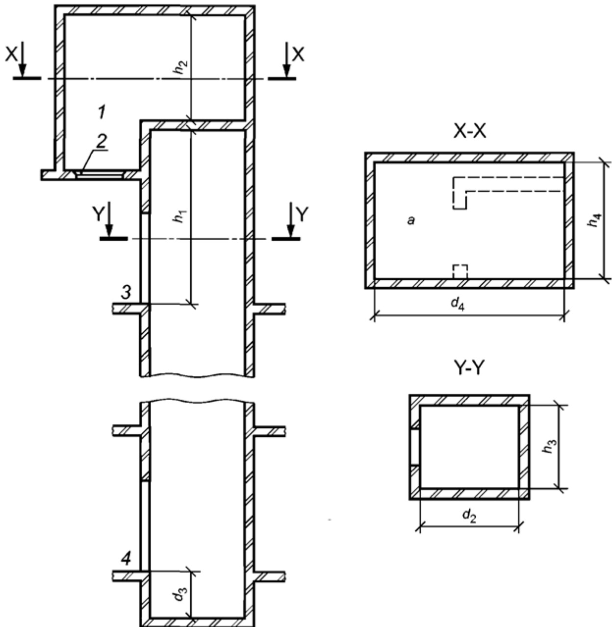
Рисунок 1 - Пассажирские лифты. Обозначение размеров кабины и дверного проема
